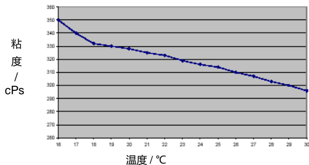
粘度 - 温度曲线
