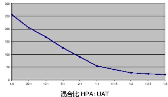
粘度曲线 (HPA: UAT)
